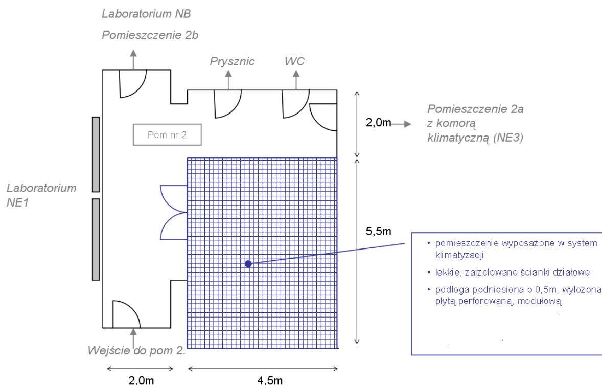
Rys.1. Schemat lokalizacji komory klimatycznej w pomieszczeniu nr 2 (przybliżone wymiary)
