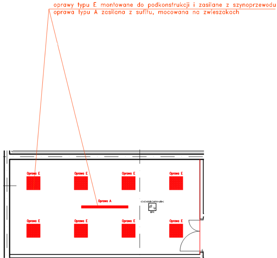
Rys. 1 Rozmieszczenie opraw oświetleniowych w pomieszczeniu 247 (laboratorium)
