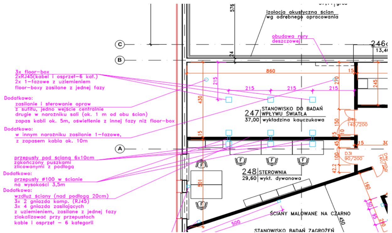
Rys. 2 Plany konstrukcyjne pomieszczeń 247 (laboratorium) i 248 (sterownia) odnośnie przeprowadzenia okablowania
